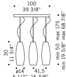
PERONI S14L 3x70W E27 alogeno chiara clear halogen 3x50W E27 - PAR 20 3x23W E27 fluorescente fluorescent
