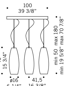
PERONI S16L 3x70W E27 alogeno chiara clear halogen 3x75W E27 - PAR 30 3x23W E27 fluorescente fluorescent
